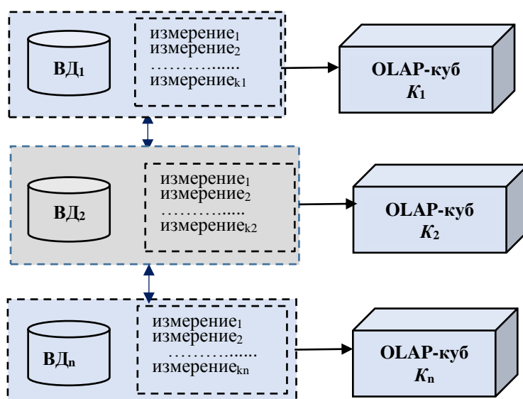
Рис. 3. Поликубическая OLAP-модель, входящая в э-демографическую СППР
