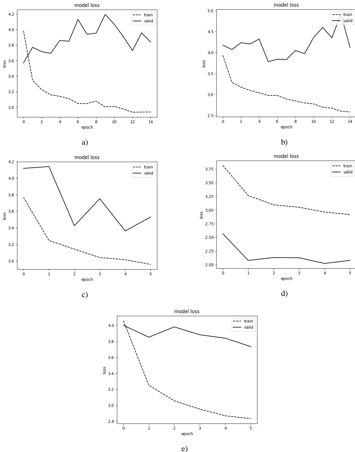
Рис. 2. Середній квадрат помилки для передісторії різної тривалості
