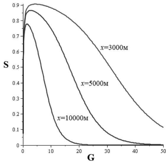
Рис.7. Графіки залежності ПЗ каналу БПЛА-БПЛА (БПЛА-МА) від інтенсивності трафіку при різних значеннях відстані між вузлами (при N=10 )
